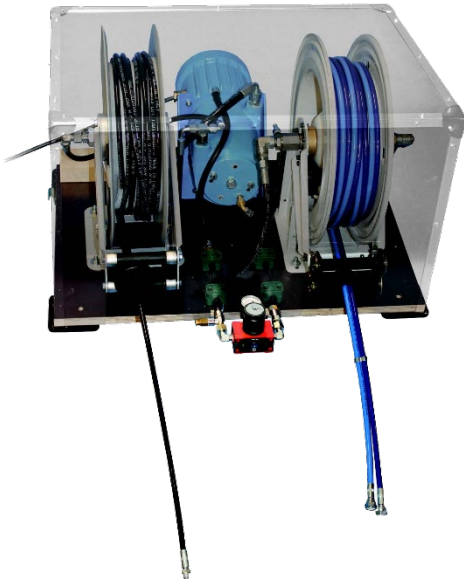
ISOLERET BOX TIL MONTERING AF SLANGEOPRULLER/PRODUKTVARMER
